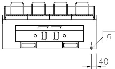
Front aanzicht
