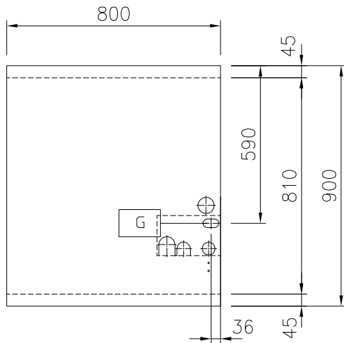
Boven aanzicht
